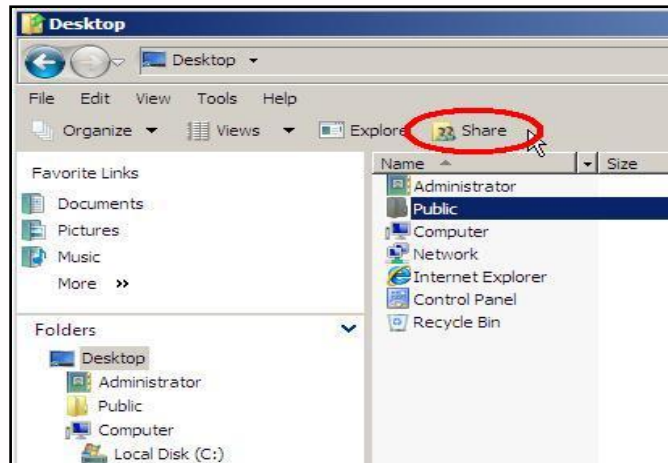
Gambar 7. 44 : Konfigurasi Sharing
