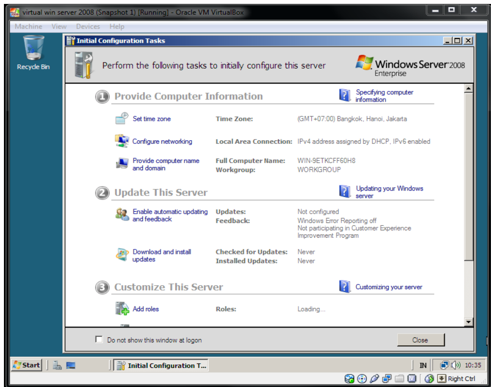
Gambar 7. 14 : Konfigurasi Awal
