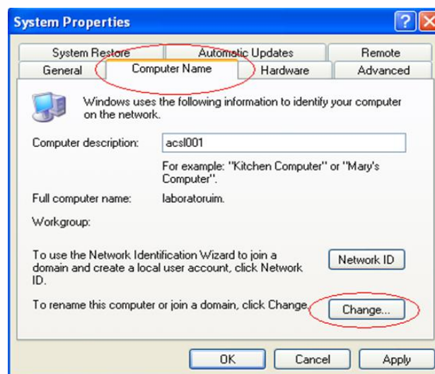
Gambar 7. 41 : Pemilihan Properties
