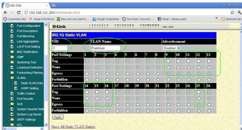
Gambar 4.23 Konfigurasi Grup VLAN (VID 3, VLAN Name Praktikan, Port 9-16 & 25)
